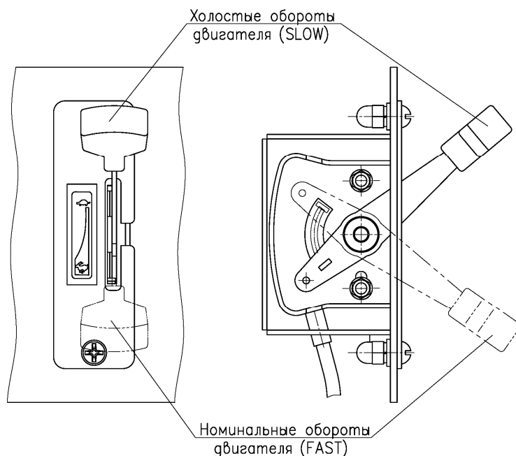
Рисунок 2 – Рычаг управления дроссельной заслонкой двигателя
