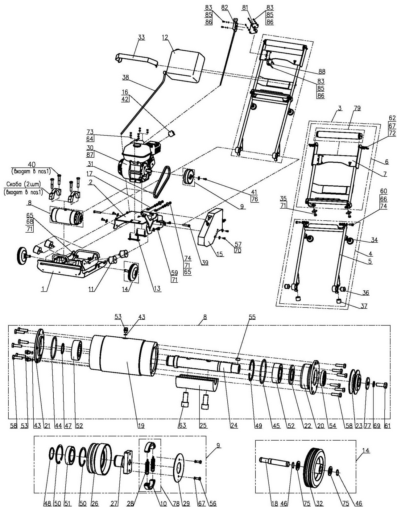
Рисунок 9 – Компоновка виброплиты
