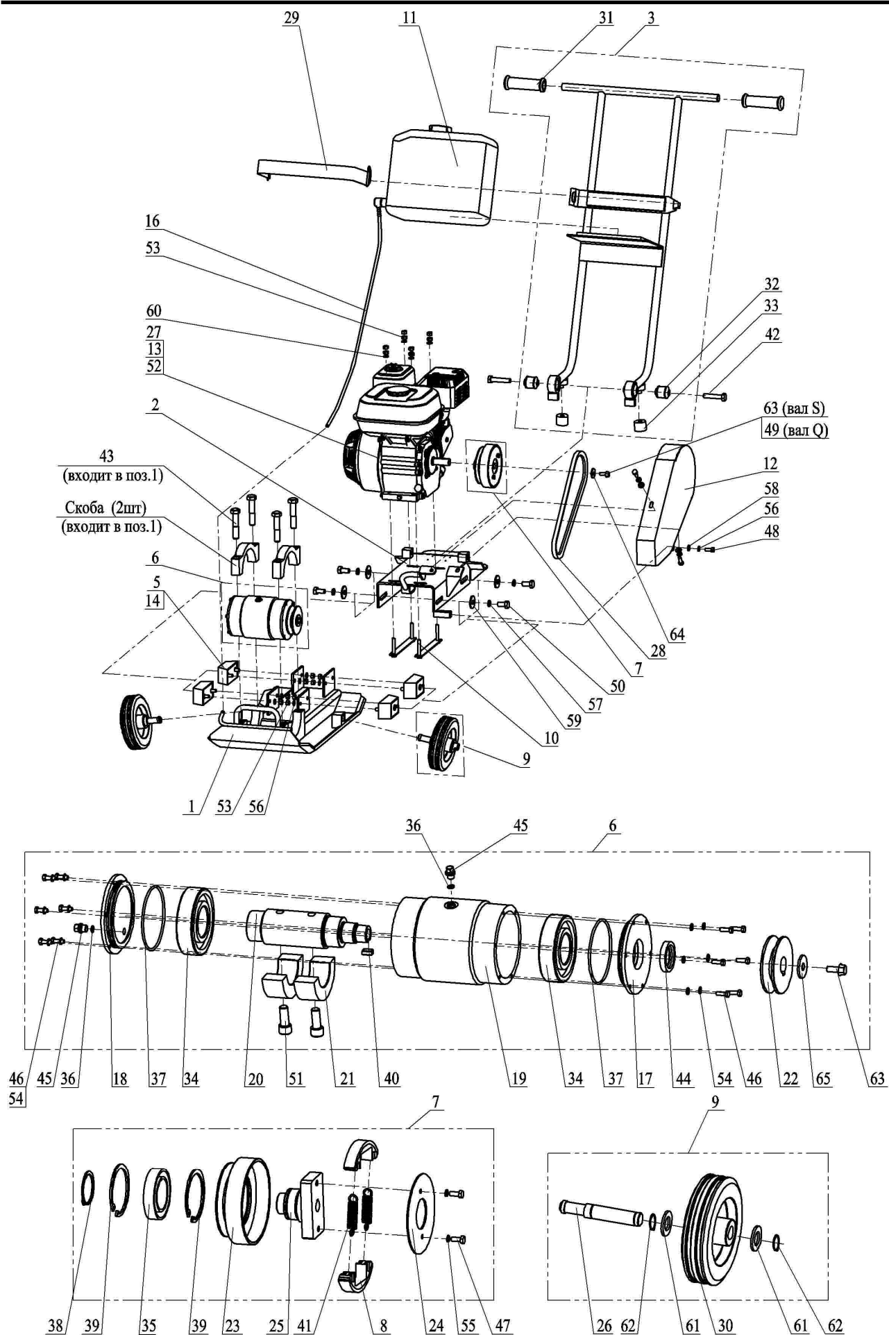
Рисунок 8 – Компоновка виброплиты
