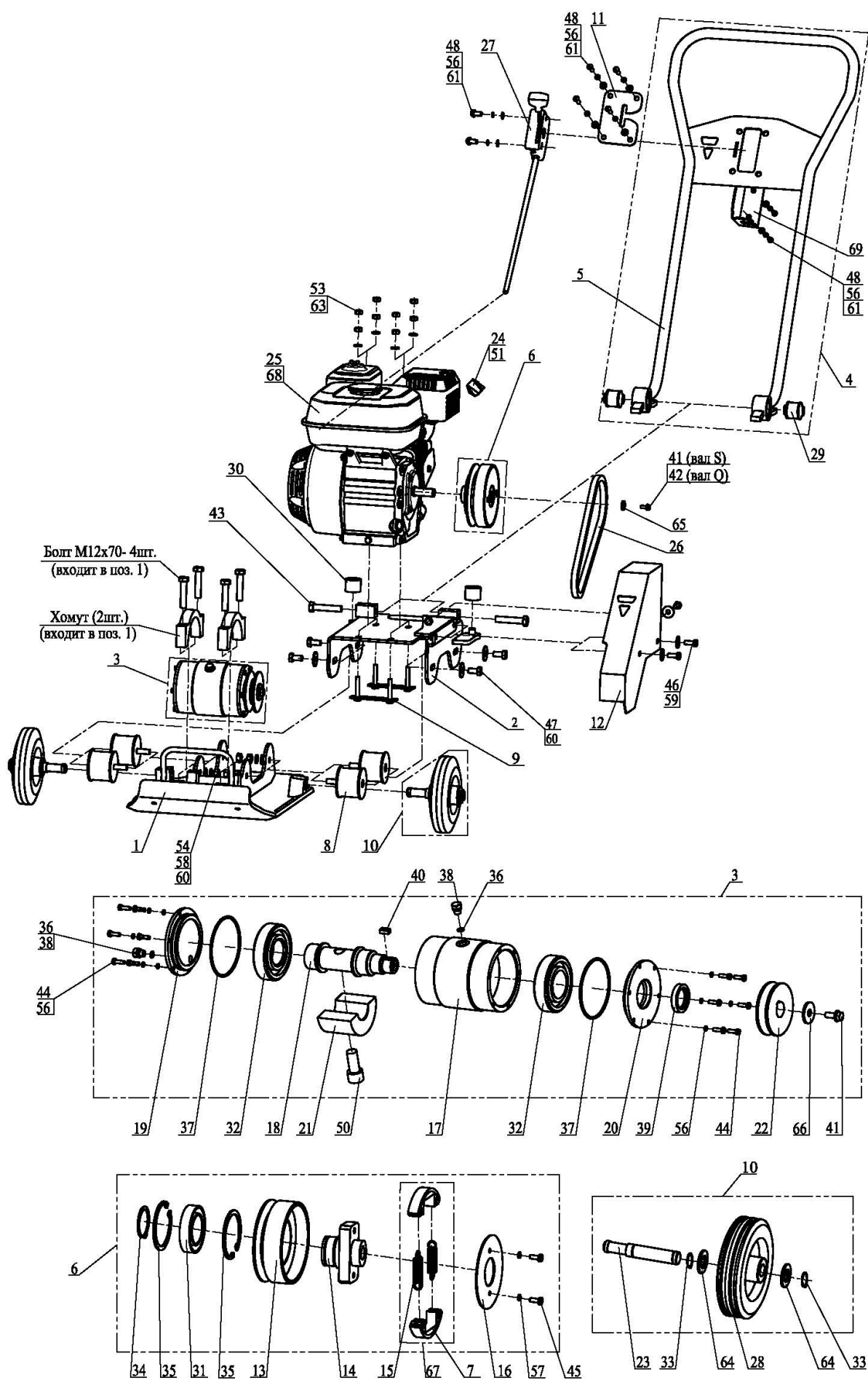
Рисунок 9 – Компоновка виброплиты
