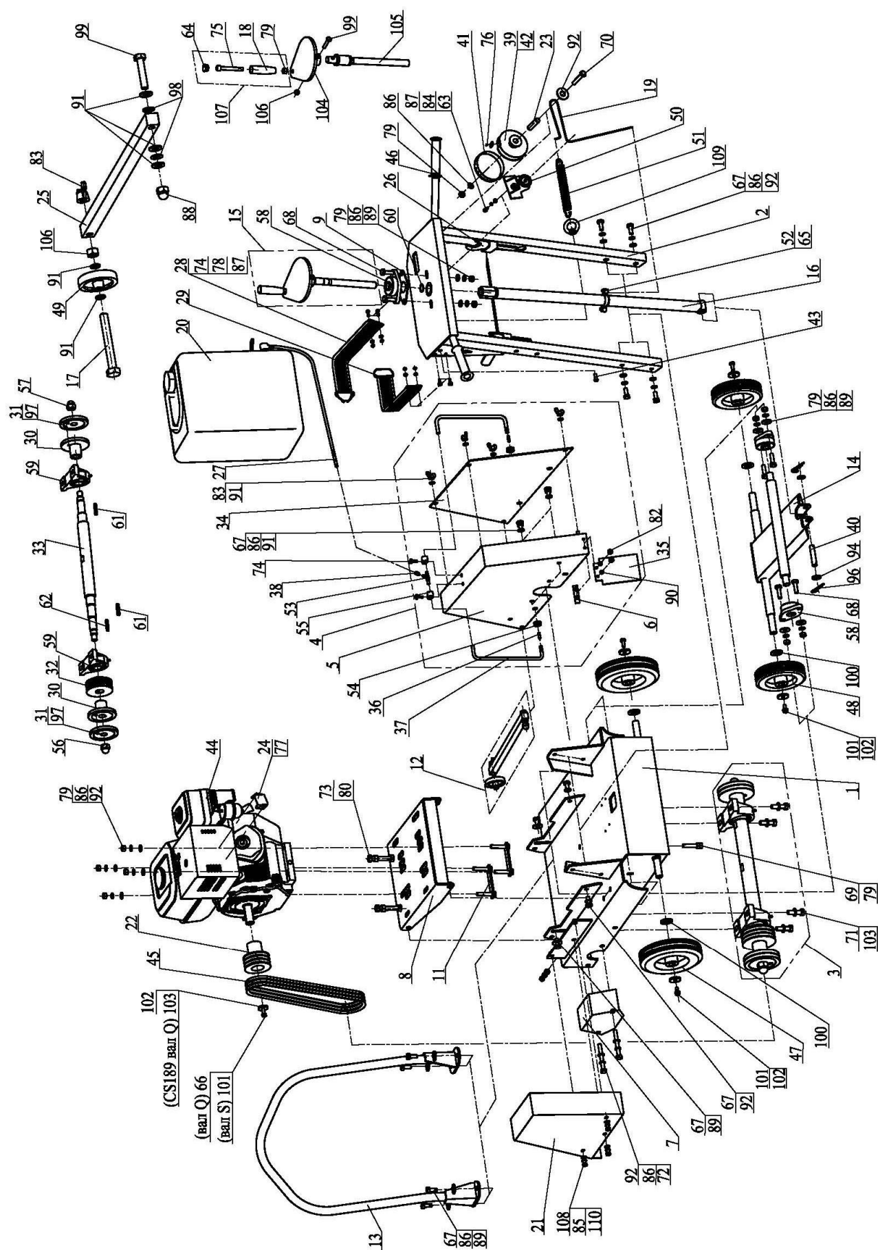
Рисунок 14 – Компоновка резчиков
