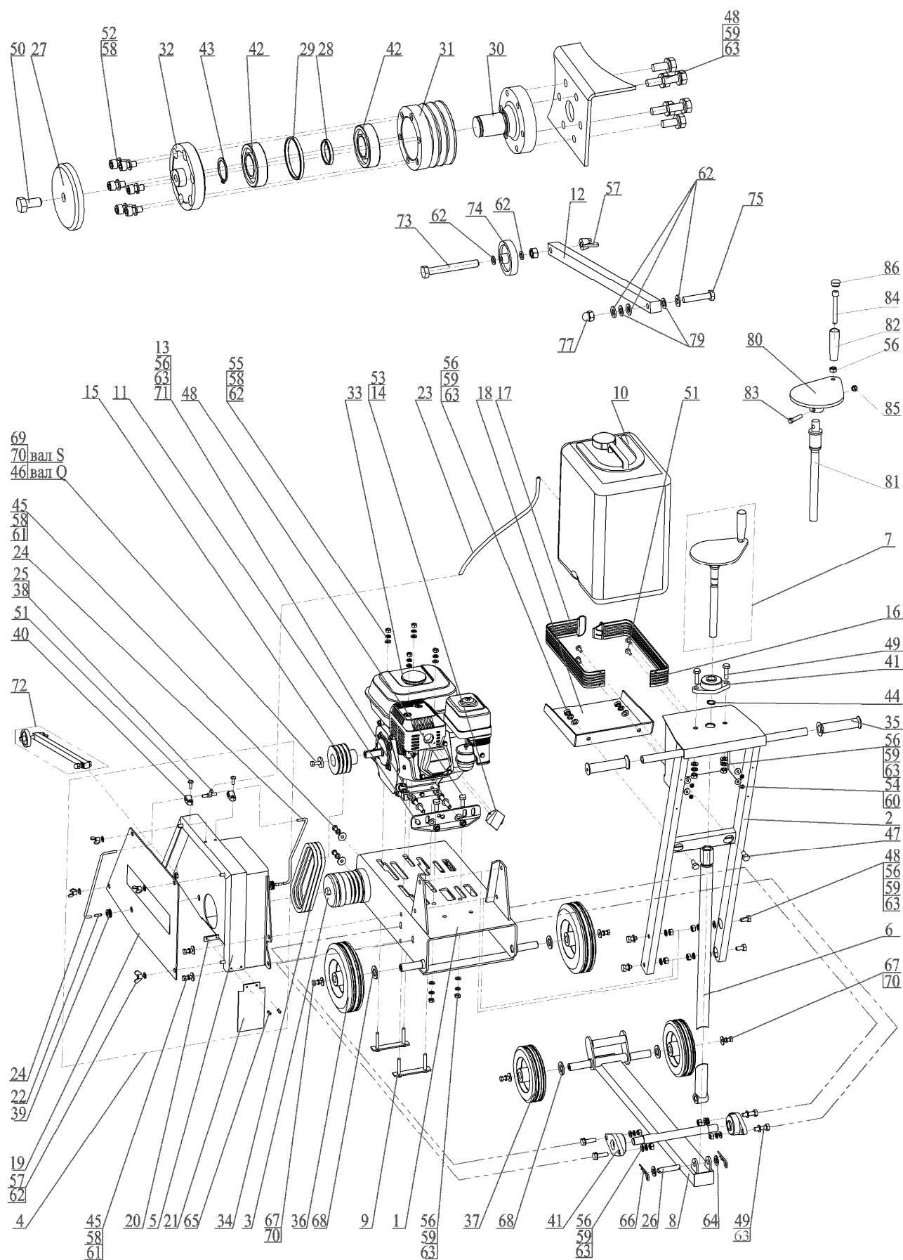
Рисунок 11 – Компоновка резчиков
