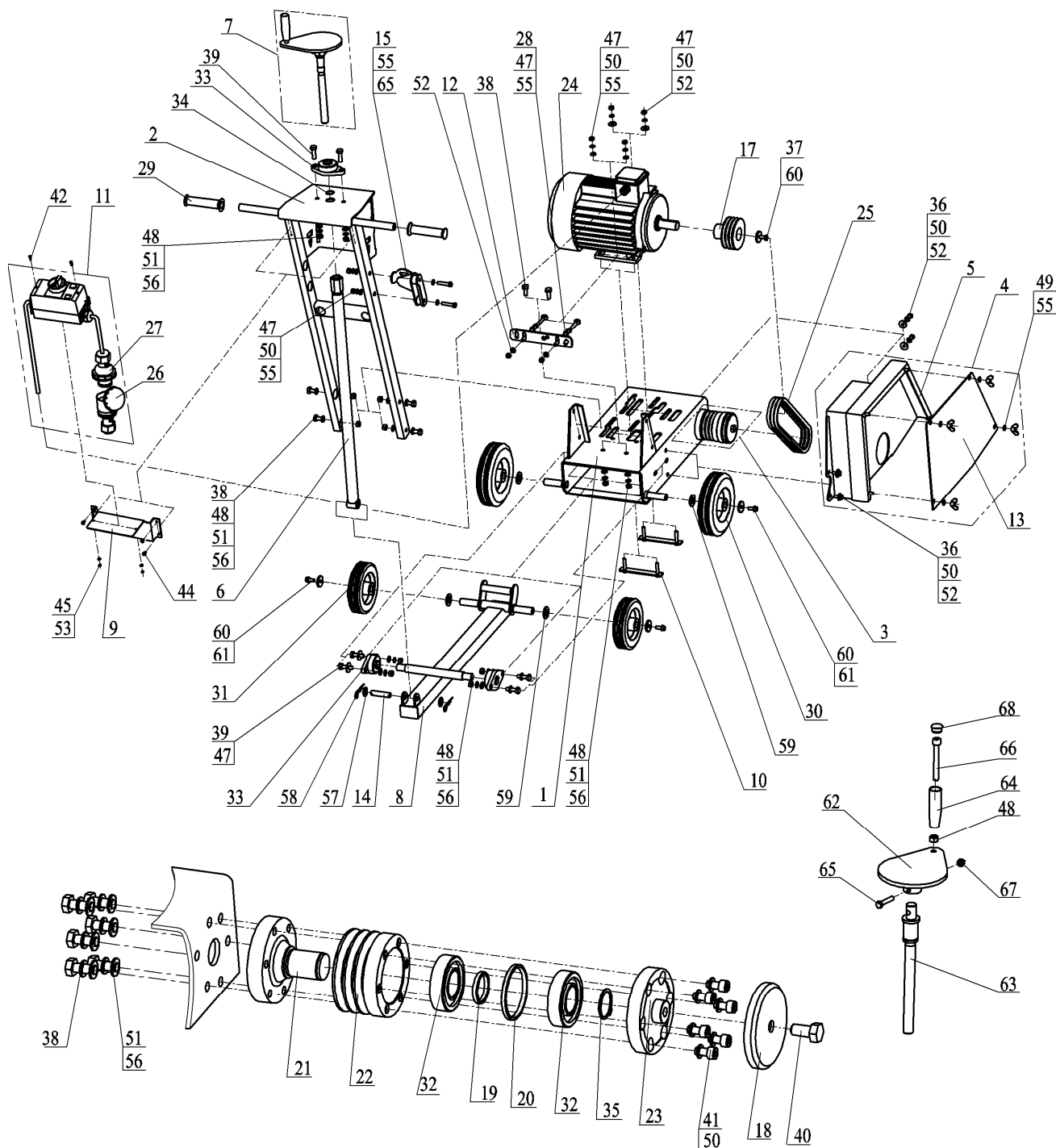
Рисунок 13 – Компоновка резчиков
